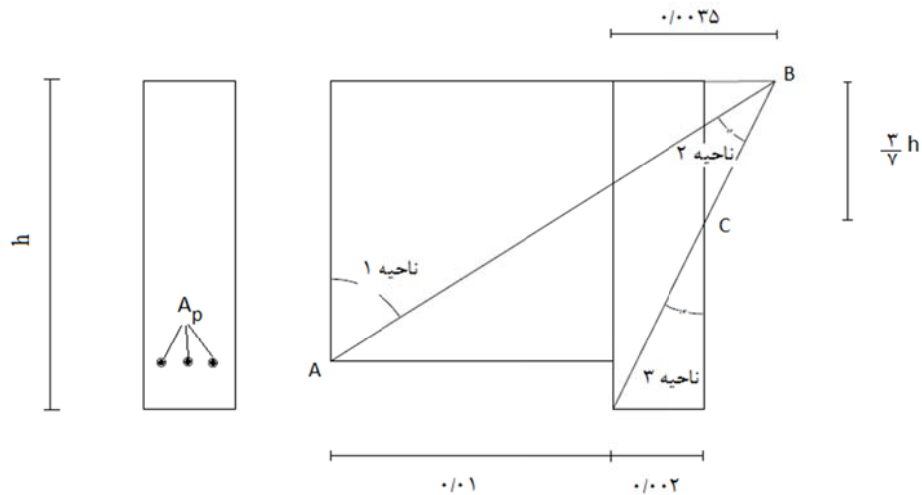
شکل ۹-۲۴-۱ نمودار تغییر شکل در حالت حدی نهایی
