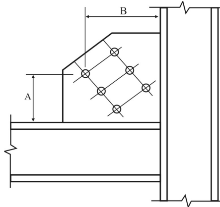
شکل ۱۴-۴-۱۰ رواداری مختصات سوراخ پیچ‌ها
