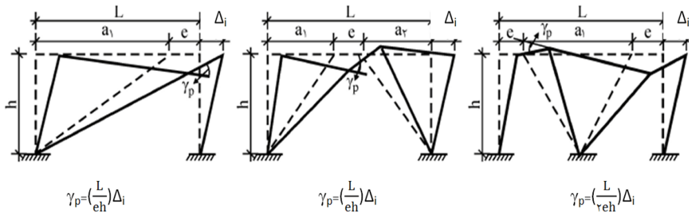
شکل ۱۰-۳-۱۲ دوران غیرالاستیک تیر پیوند نسبت به ناحیه خارج از آن ( \gamma_p )
