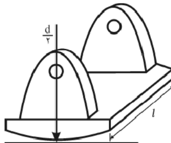
شکل ۱۴-۹-۲-۱۰ کفشک‌های تکیه‌گاهی
