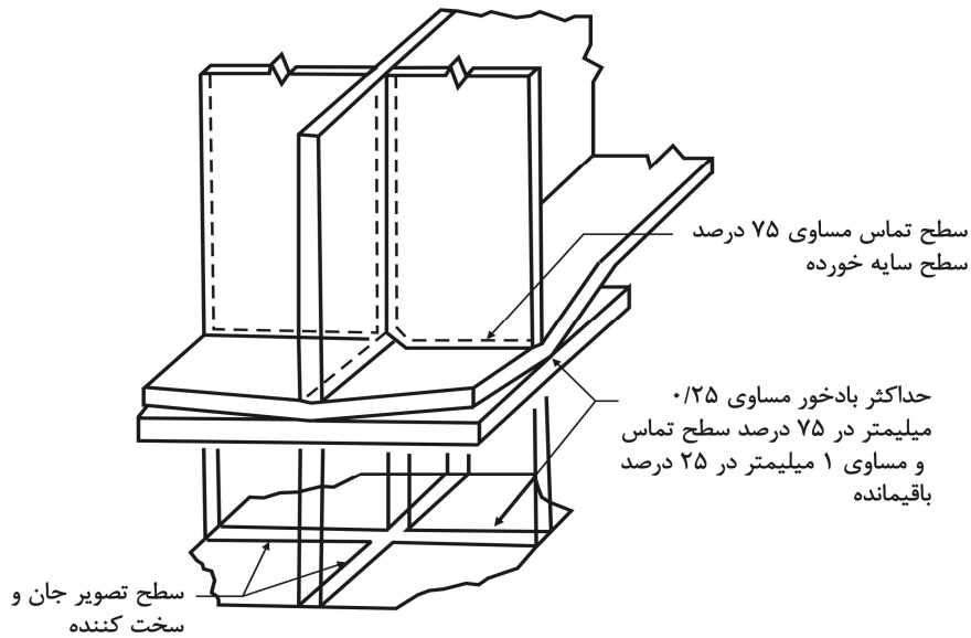
شکل ۱۰-۴ رواداری در محل تماس تیر با تکیه گاه - تیر با سخت کننده تکیه گاهی
