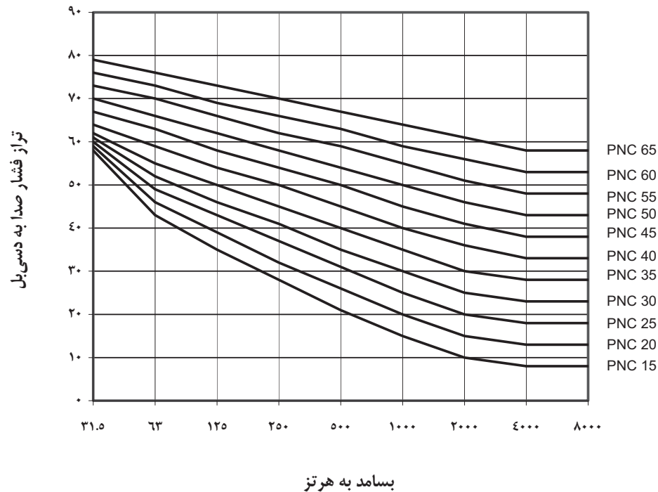
شکل ۱۸-۳-۴: نمودارهای پرسنج ترجیحی نوفه PNC
